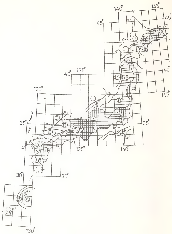
Fig. 5.1 Seismic Zoning
